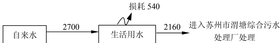
图 5-2 全厂水平衡图 (t/a)
