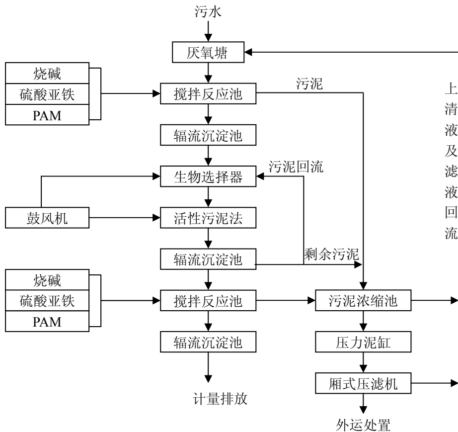
图 8-1 污水厂污水处理工艺流程图
