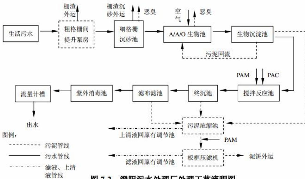
图 7-2 澄阳污水处理厂处理工艺流程图
