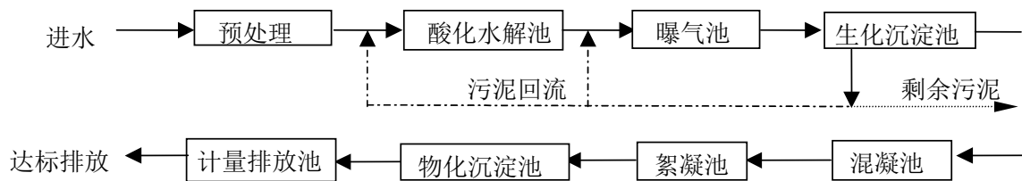
图 8 污水处理厂污水处理工艺流程图
