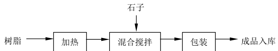
图 5 透水砂石生产工艺流程图
