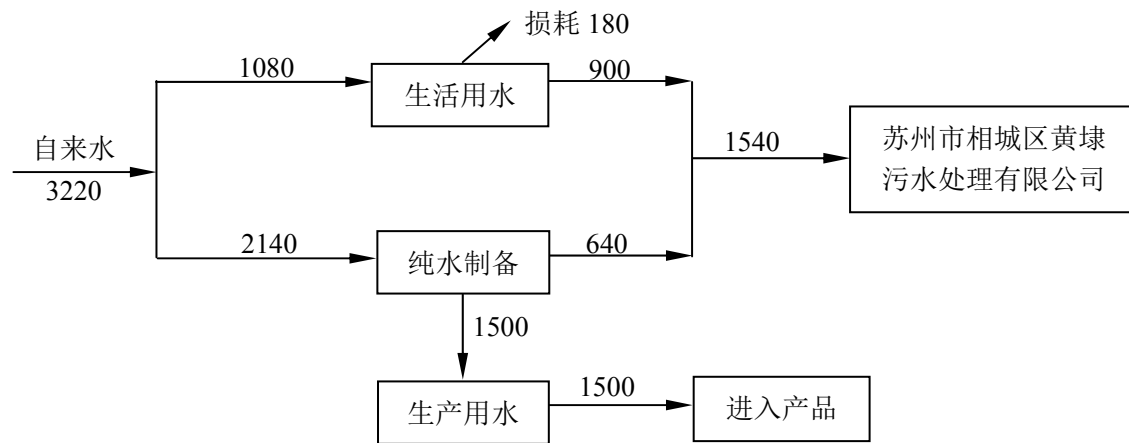
图 7 全厂水平衡图 (t/a)
