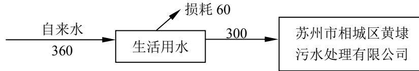
图 6 本项目水平衡图 (t/a)
