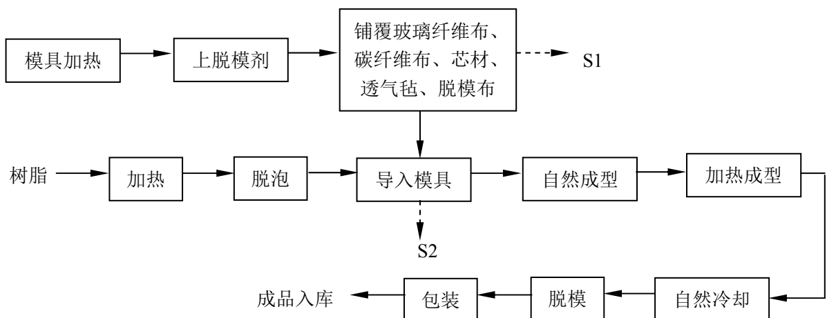
图 4 太阳能和风力发电配件等生产工艺流程（不规则配件）
