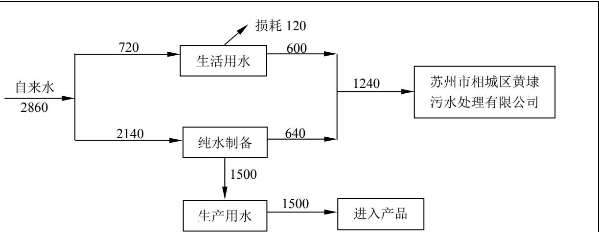
图 2 现有项目水平衡图 (t/a)
