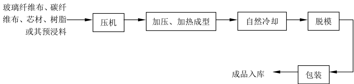
图 3 太阳能和风力发电配件等生产工艺流程（规则配件）
