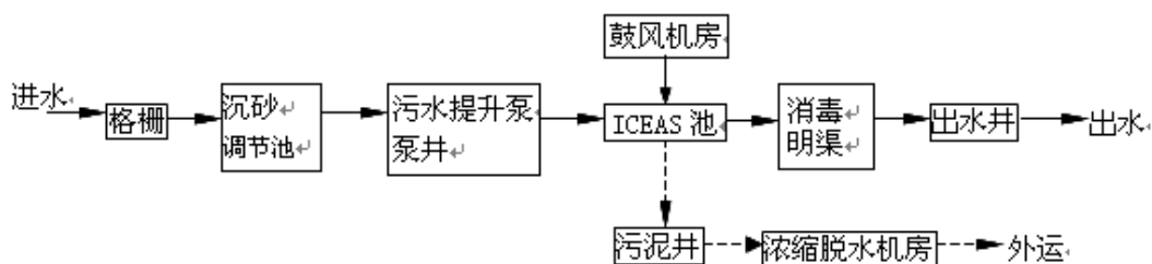
图 7-1 污水厂污水处理工艺流程图
